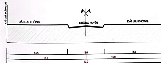
MẶT CẮT 1-1
